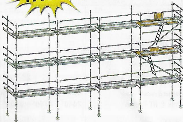
Version avec lisses
